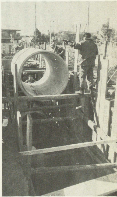
急ピッチで進む下水道工事
